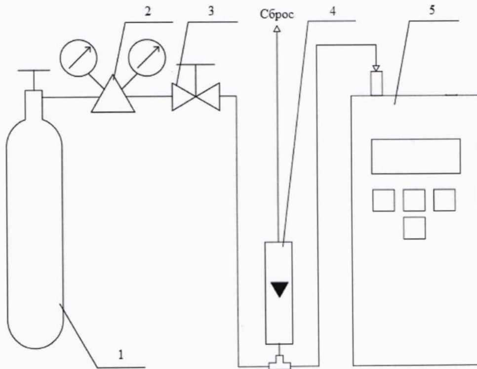
1 – баллон с ГС; 2 – редуктор баллонный; 3 – вентиль точной регулировки трассовый; 4 – ротаметр (индикатор расхода); 5 – поверяемый газоанализатор (показан условно).
